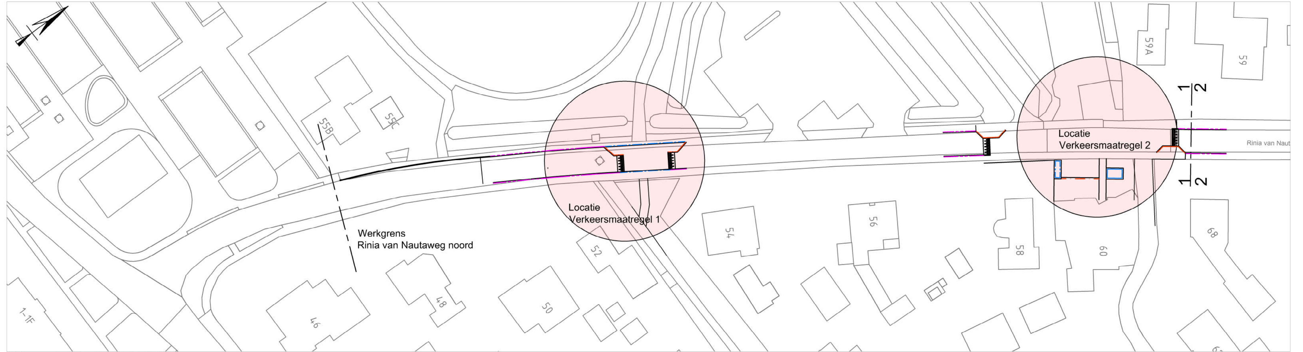
Situatie 1-1 1:500
